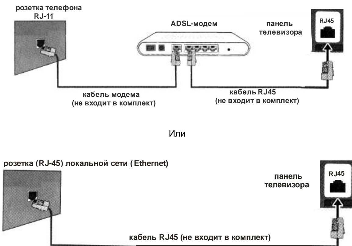
Рисунок 8 – Проводное подключение
